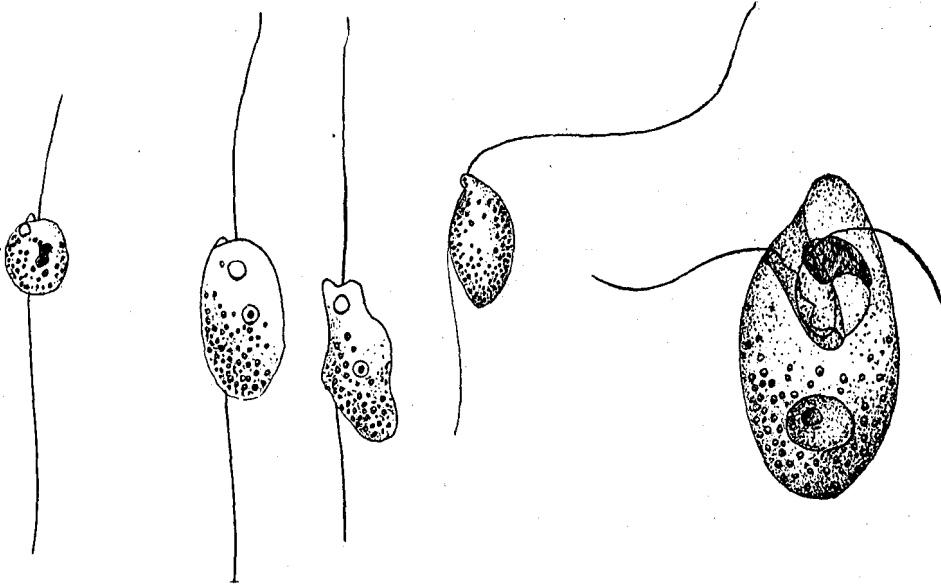
FIG. 14.— Bodo caudatus .
