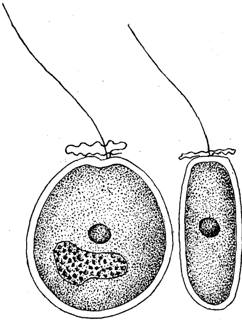
FIG. 18.— Exuviella lima .
