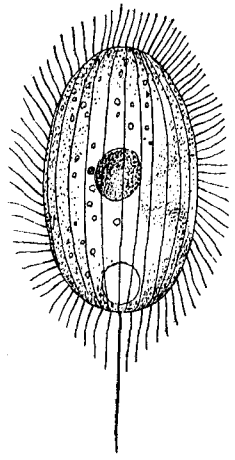
FIG. 39.— Uronema marina .
