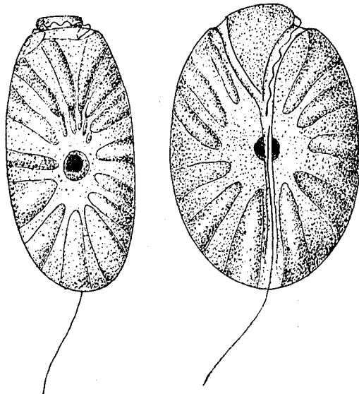
FIG. 27.— Amphidinium operculatum .
