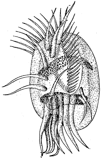
FIG. 54.— Diophrys appendiculatus .
