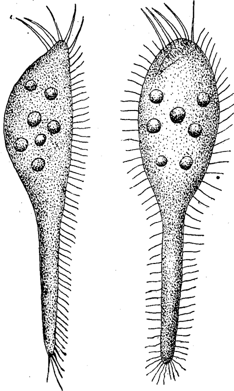
FIG. 50.— Epiclintes radiosa .
