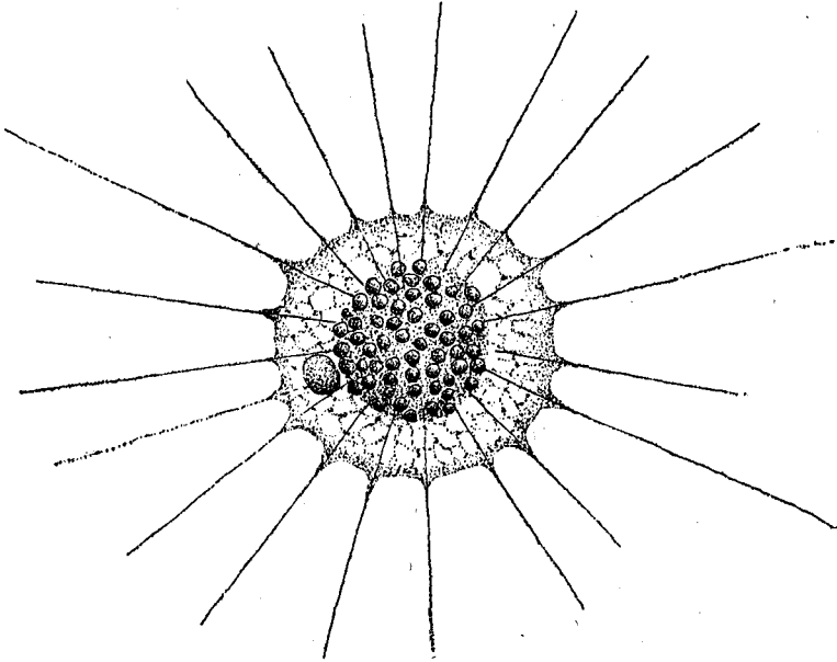
FIG. 6.— Heterophrys myriapoda .
