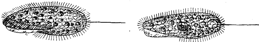
FIG. 43.— Lencbus pusillus .
