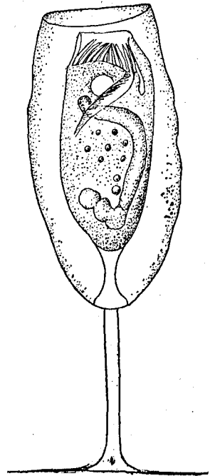
FIG. 64.— Cothurnia nodosa .
