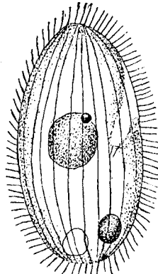
FIG. 38.— Colpidium colpoda .
