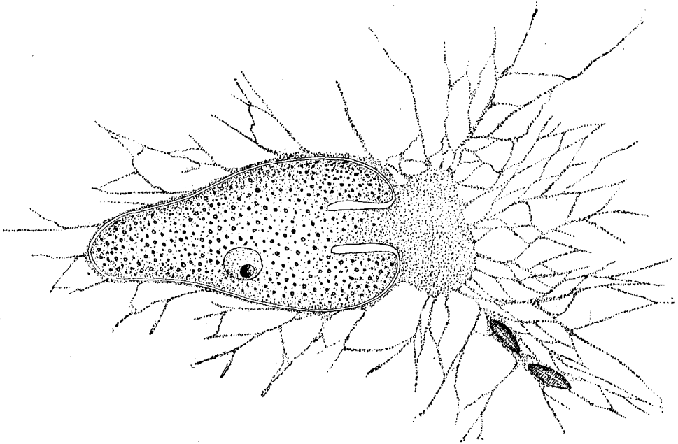
FIG. 4.— Gromia lagenoides .
