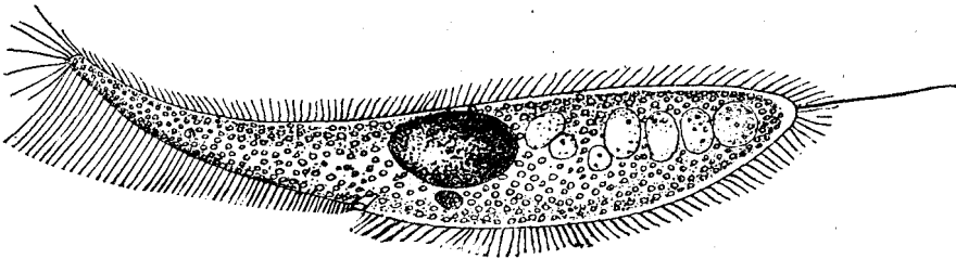
FIG. 42.— Lembus infusionum .
