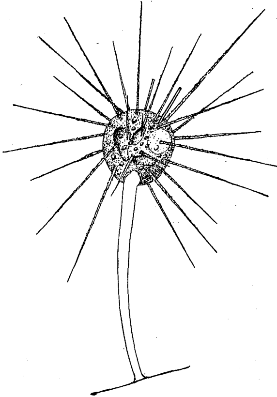
FIG. 66.— Ephelota coronata .
