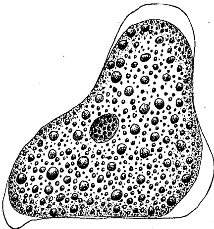
FIG. 2.— Amœba sp.
