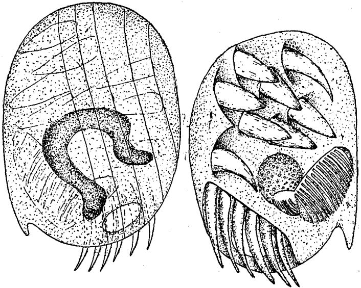
FIG. 56.— Aspidisca hexeris .
