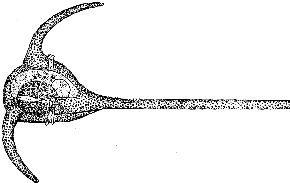
FIG. 25.— Ceratium tripos .
