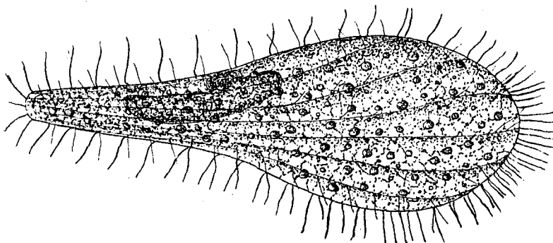
FIG. 44.— Anoplophrya branchiarum .
