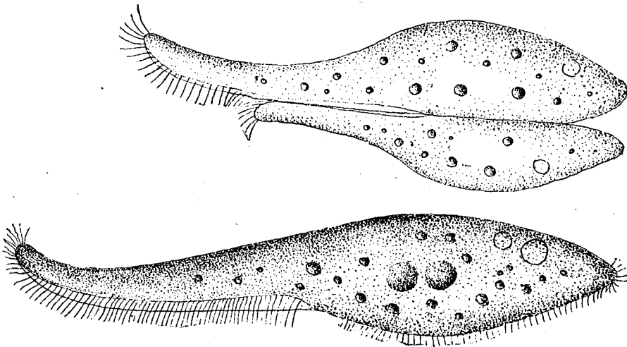
FIG. 33.— Lionotus fuscicola .
