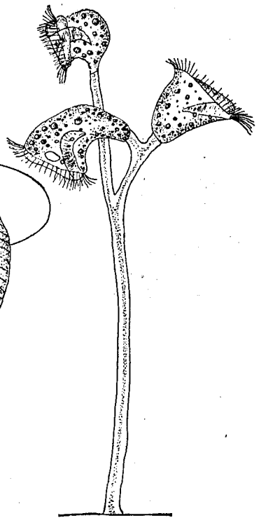
FIG. 61.— Zoothamnium elegans .
