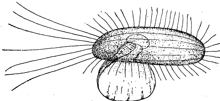
FIG. 41.— Pleuronema setigera .
