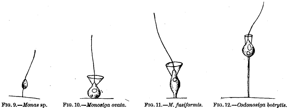
FIG. 9.— Monas sp.
