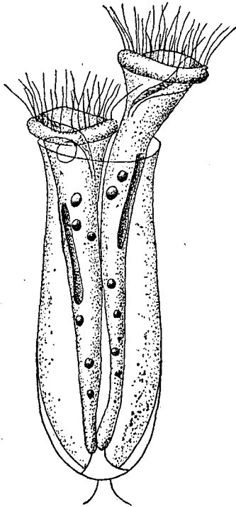
FIG. 63.— Cothurnia imberbis .
