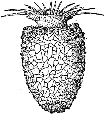
FIG. 47.— Tintinnopsis beroidea .
