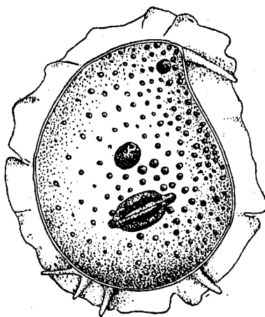
FIG. 3.— Trichosphaerium sicboldi .
