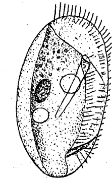
FIG. 36.— Dysteria lanceolata .
