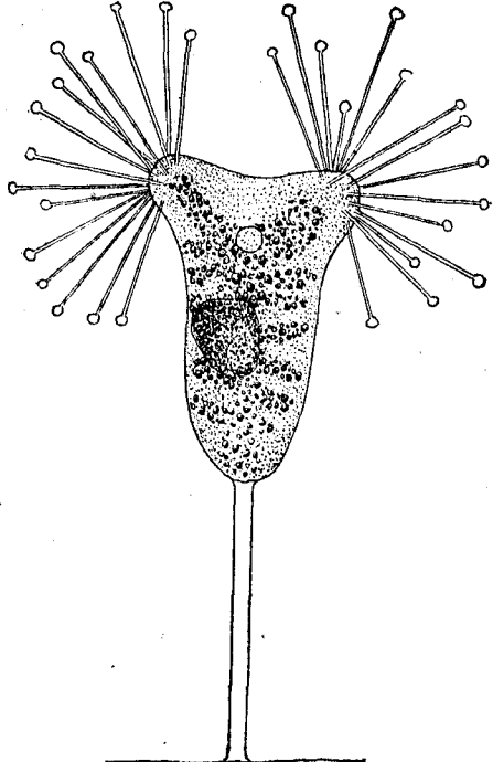
FIG. 68.— Acineta tuberosa .
