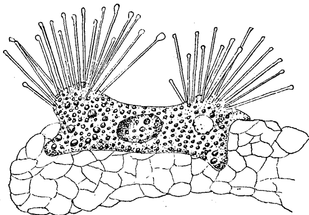
Fig. 69.— Trichophrya salparum .
