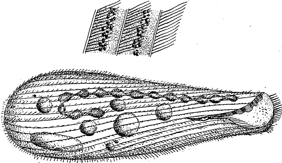
FIG. 45.— Condylostoma patens .
