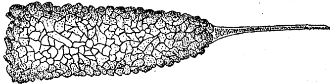
FIG. 48.— Tintinnopsis davidoffi .
