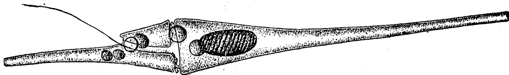
FIG. 26.— Ceratium fusus .
