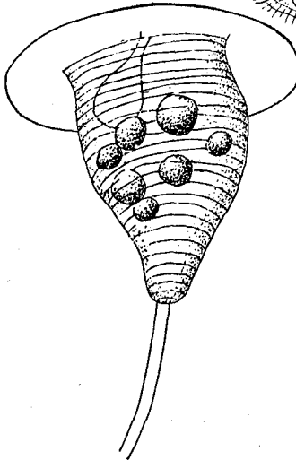
FIG. 60.— Vorticella marina .
