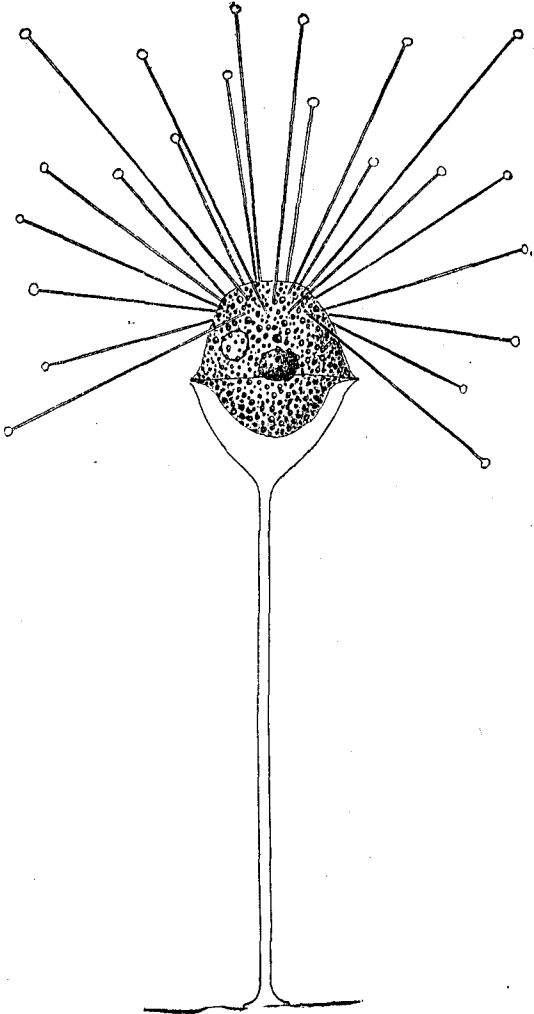
FIG. 67.— Acineta divisa .
