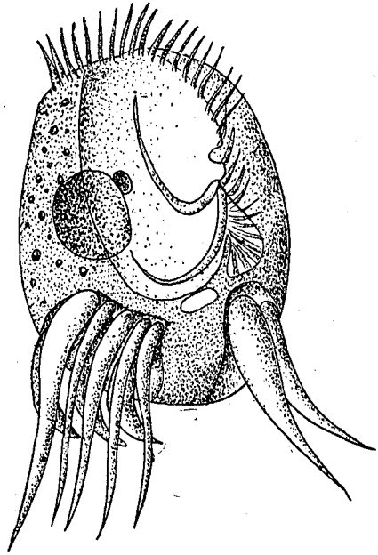
FIG. 55.— Uronychia setigera .
