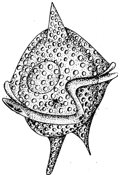
FIG. 23.— Peridinium digitale .
