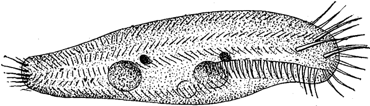
FIG. 51.— Amphisia kessleri .
