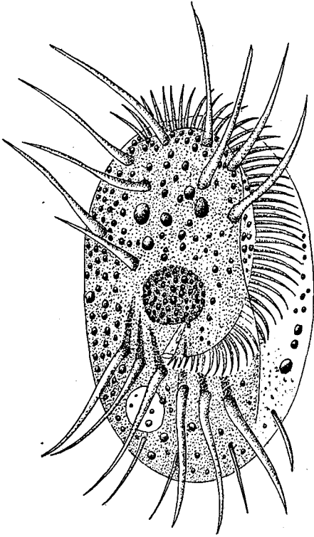
FIG. 53.— Euplotes harpa .
