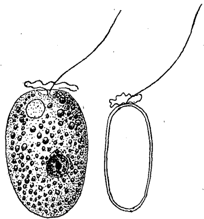
FIG. 19.— Exuviella marina .
