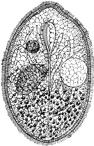
FIG. 37.— Frontonia leucas .
