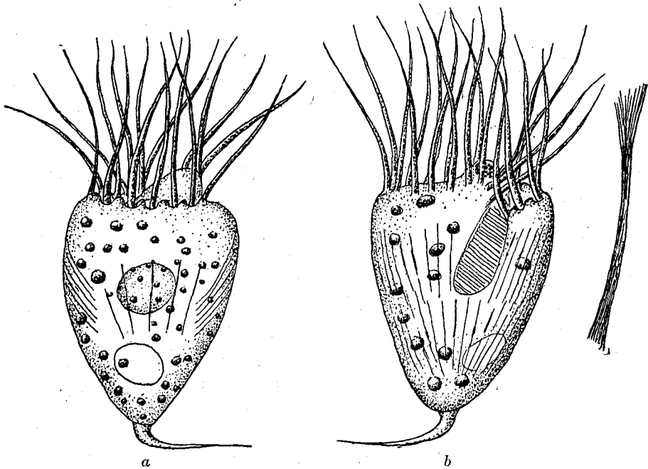
FIG. 46.— Strombidium caudatum .
