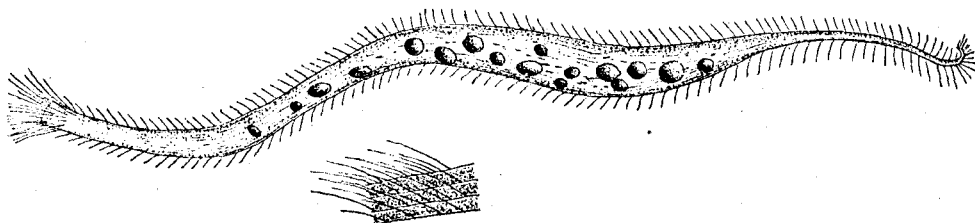
FIG. 30.— Trachelocerca phanicopterus .
