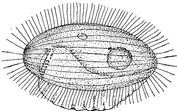
FIG. 40.— Pleuronema chrysalis .
