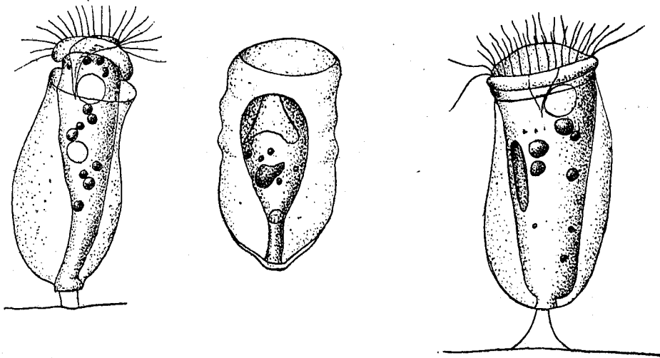
FIG. 62.— Cothurnia crystallina .
